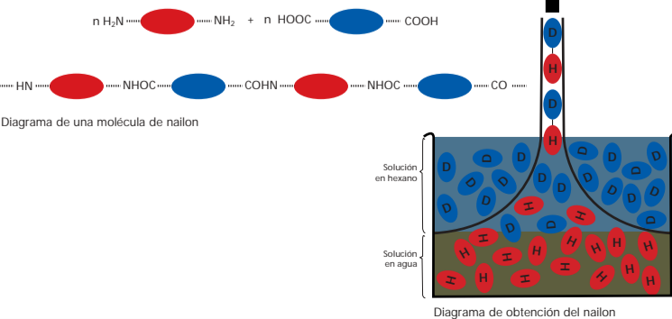
Diagrama de obtención del nailon
